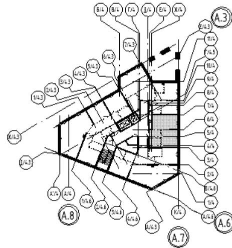
Схема расположения квартир на 2 этаже
