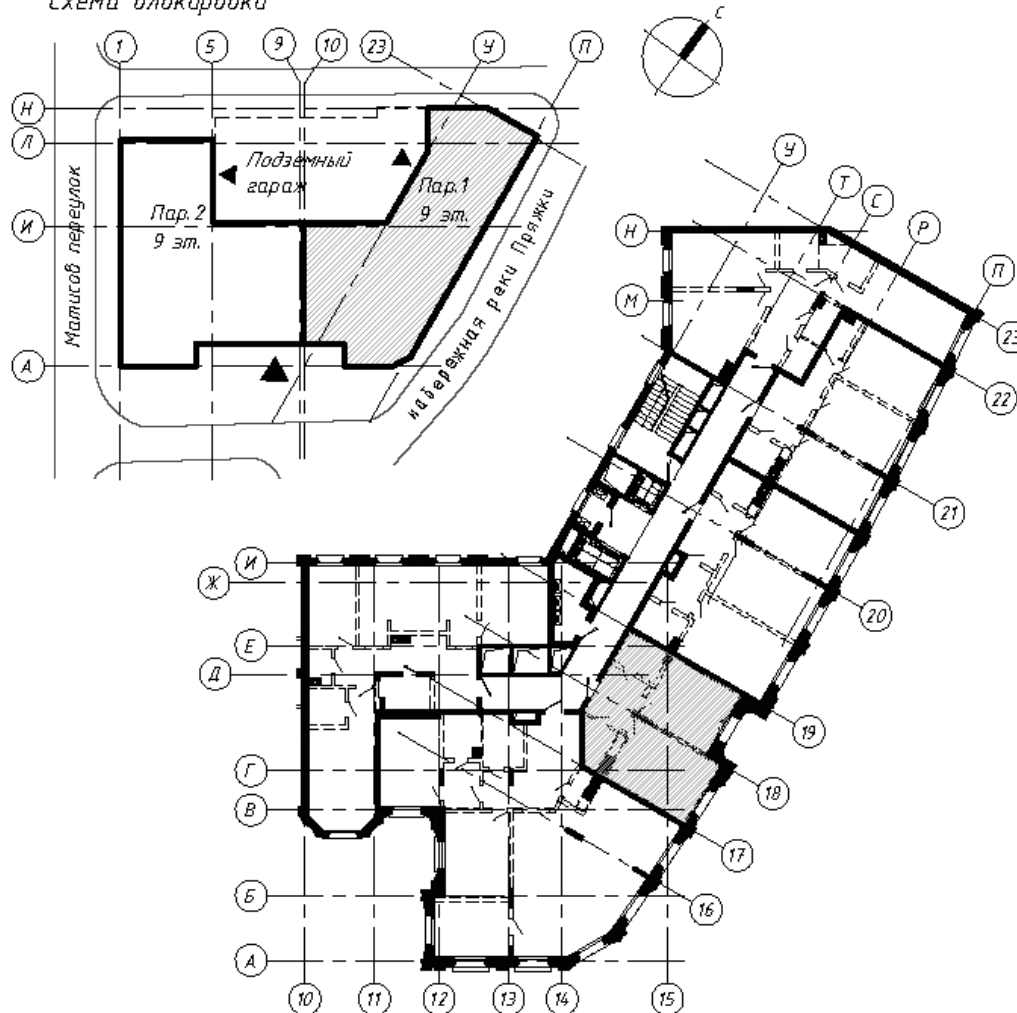
Схема блокировки
