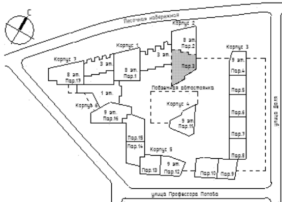
Схема блокировки
