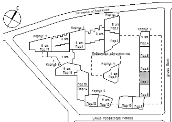
Схема блокировки
